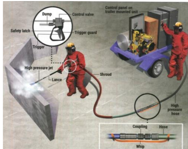
Figura 10 – Distanciamento Hidrojetista e Operador (Vigia).
