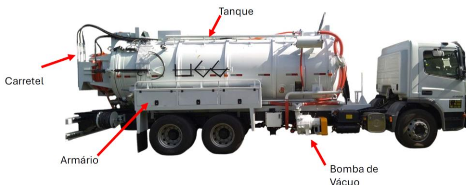
Figura 02 - Caminhão Combinado – Vista bomba de vácuo
