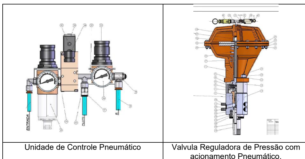
Figura 04 – Válvula reguladora de pressão e controle pneumático.
